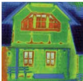
PRIMA DEL MONTAGGIO: VECCHIE FINESTRE
